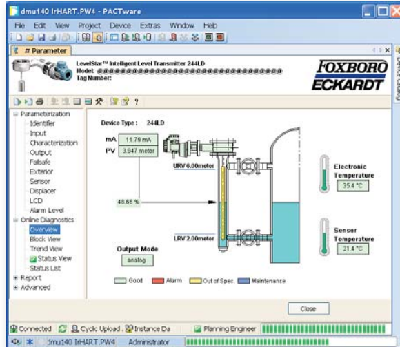
PACTware: Operation
